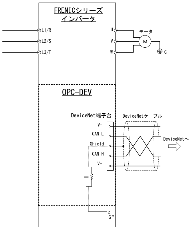
図 4.1 基本接続図
