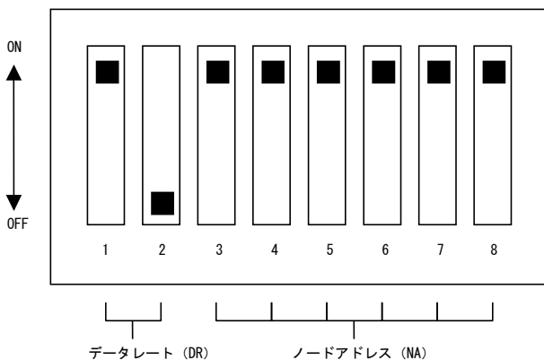
図 2.2 DIP スイッチ詳細 (図はデータレート 500kbps、ノードアドレス 63)
