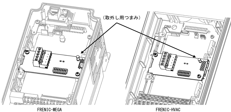
図 3.3 取付け完了（B-port 取付け時）
