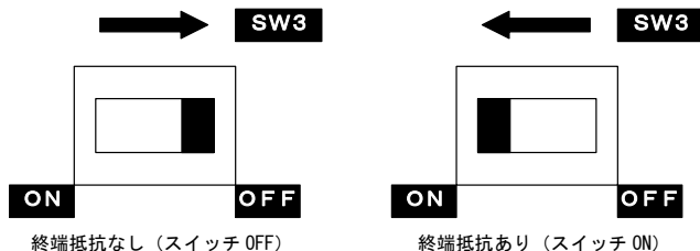
図 2.3 終端抵抗 ON/OFF スwitchの設定
