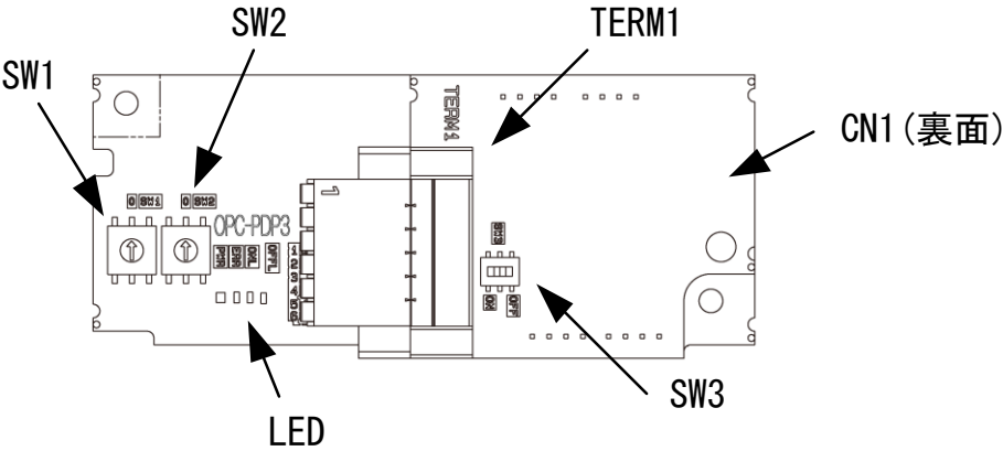
図 2.1 OPC-PDP3 の外観
