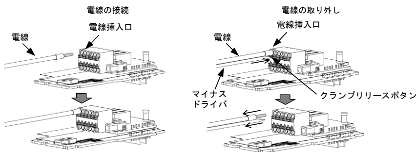
図 4.2 PROFIBUS ケーブル電線の接続と取り外し
