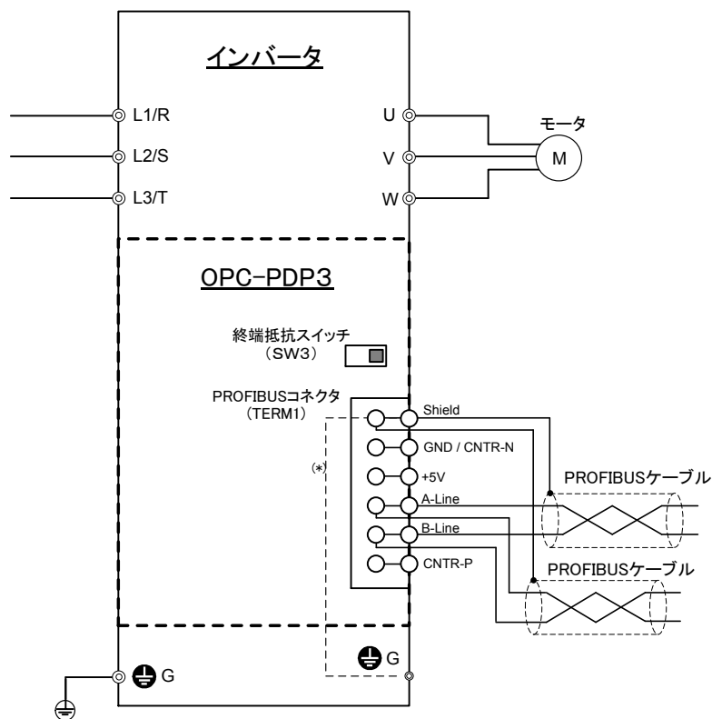
図 4.1 基本接続図
